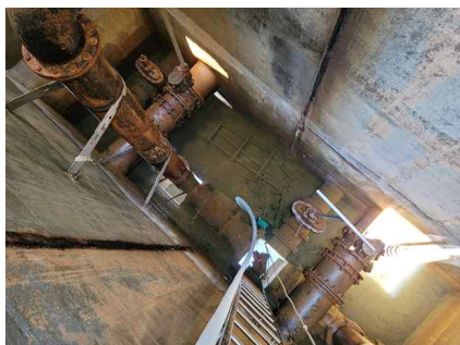
<통합유출밸브실 바닥슬래브 채수>
