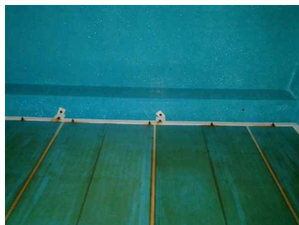
<배수지 1지 도류벽 브라켓 파손>
